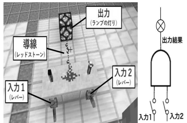
図 1 Minecraft 内で作成した AND 回路
